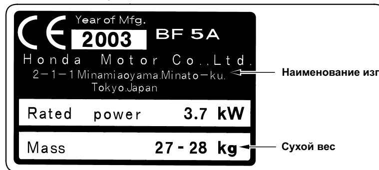
СЕРТИФИКАЦИОННАЯ ТАБЛИЧКА
