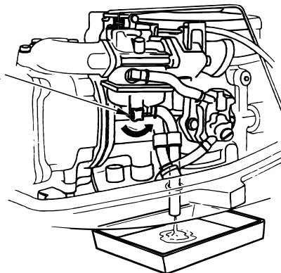
СЛИВНАЯ ПРОБКА
