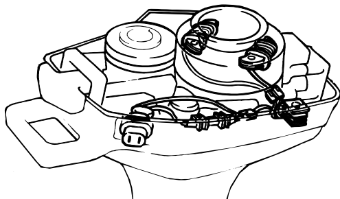
КОМПЛЕКТ СТАТОРНЫХ ОБМОТОК ДЛЯ ЗАРЯДКИ АККУМУЛЯТОРА И ОСВЕЩЕНИЯ (Дополнительное оборудование, не входящее в базовый комплект продажи)
